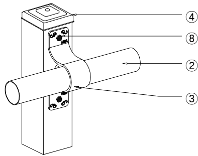
조립 상세도 SCALE : NONE
