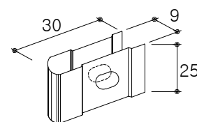
U-BAND 상세도 SCALE : NONE
