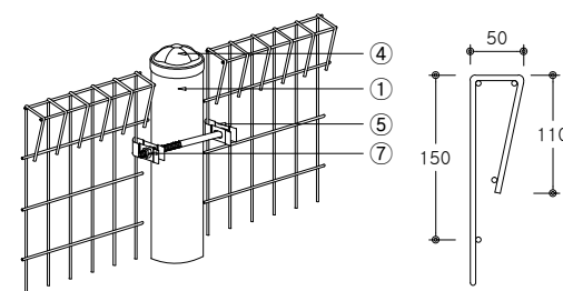
U-BAND 조립도 SCALE : NONE
