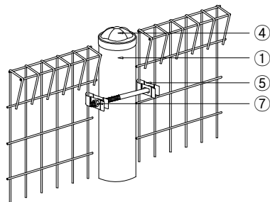
U-BAND 조립도 SCALE : NONE
