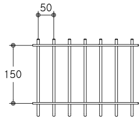
메쉬판 상세도 SCALE : NONE
