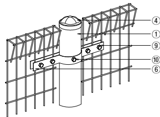
메쉬연결밴드 조립도 SCALE : NONE
