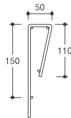
절곡 상세도 SCALE : NONE
