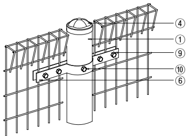
메쉬연결밴드 조립도 SCALE : NONE
