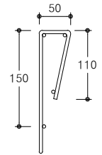
절곡 상세도 SCALE : NONE
