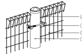
메쉬판 조립도 SCALE : NONE
