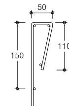
절곡 상세도 SCALE : NONE
