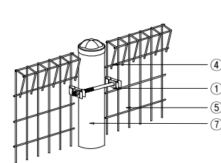
메쉬판 조립도 SCALE : NONE
