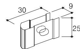
U-BAND 상세도 SCALE : NONE
