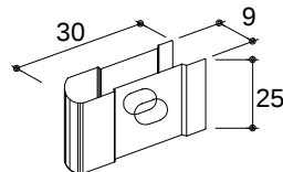
U-BAND 상세도 SCALE : NONE
