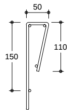
절곡 상세도 SCALE : NONE
