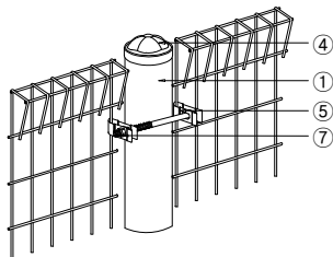
메쉬판 조립도 SCALE : NONE
