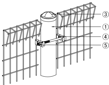
⊙ 메쉬판 조립도 SCALE : NONE
