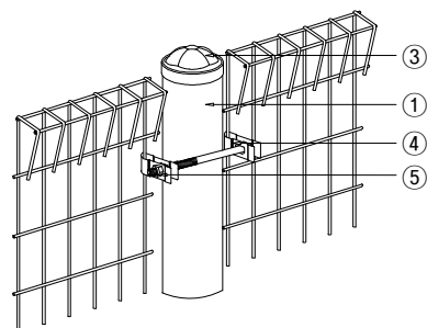
메쉬판 조립도 SCALE : NONE
