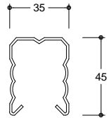
횡대 상세도 SCALE : NONE
