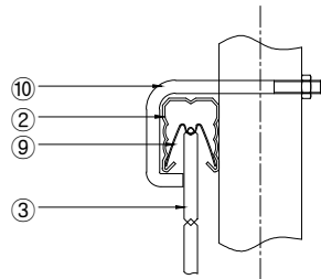
조립 상세도(상단) SCALE : NONE
