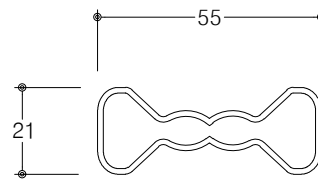
종대 상세도 SCALE : NONE
