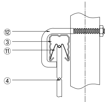
조립 상세도 SCALE : NONE
