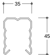
HINGE 상세도 SCALE : NONE
