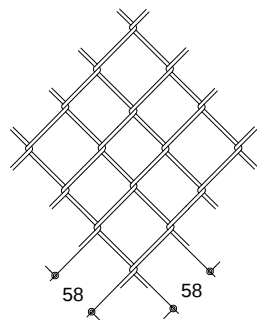
MESH 간격 상세도 SCALE : NONE
