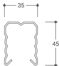
호대 상세도 SCALE : NONE
