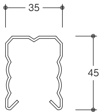
항대 상세도 SCALE : NONE
