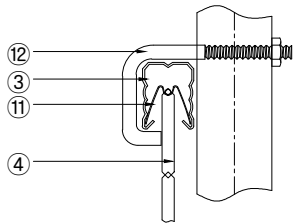
조립 상세도(상단) SCALE : NONE
