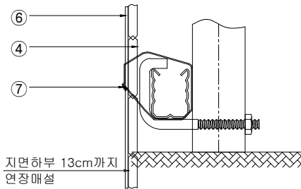
조립 상세도(하단) SCALE : NONE
