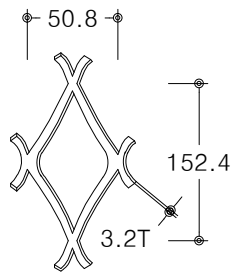
EX-메탈라스상세도 SCALE : NONE
