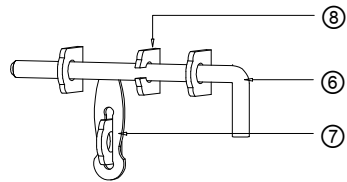
빗장상세도 SCALE : NONE
