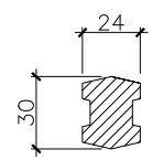
단면 "A"
